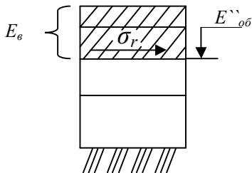
Рис. 2. Схема к расчету изгибающих напряжений в пакете асфальтобетонных слоев
