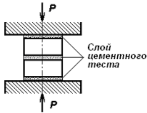
Рис. 7. Испытание кирпича на сжатие
