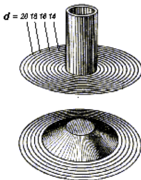
Рис. 9. Вискозиметр Суттарда
