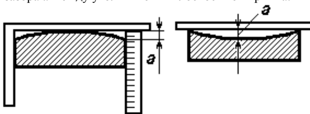
Рис. 6. Измерения отклонения геометрических размеров кирпича керамического
