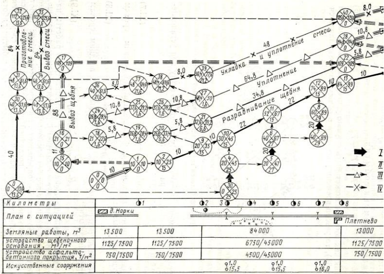
Рис. 1. Сетевой график для планирования дорожных работ: I – устройство труб; III – земляные работы; III – устройство основания; IV – устройство покрытия.
